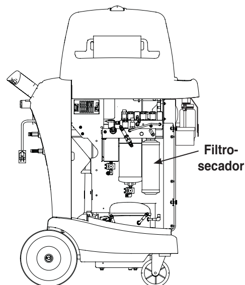
Figura 11 vista posterior sin cubierta
