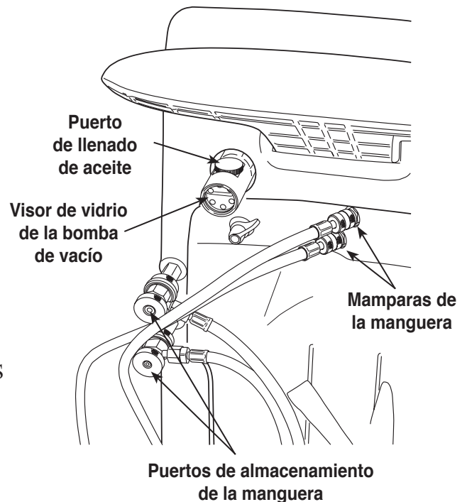
Figura 4 Vista lateral
